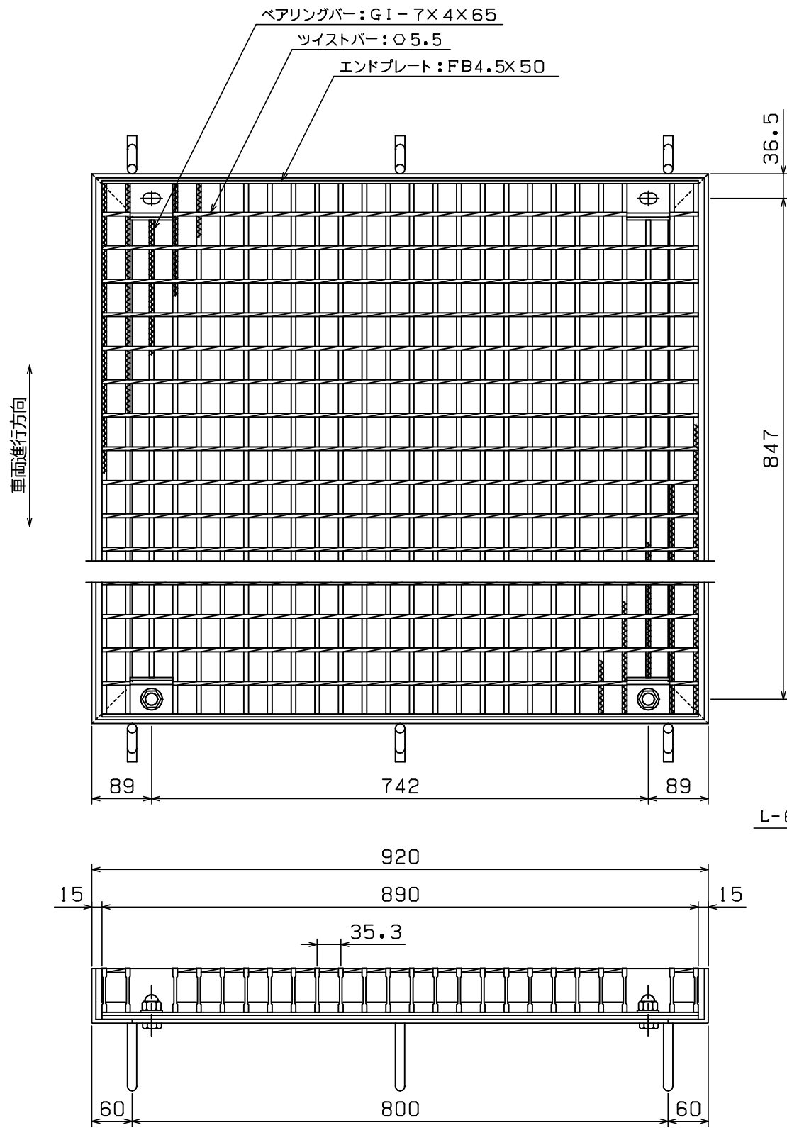
主部材ノンスリップ部詳細
