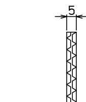
主部材ノンスリップ部詳細
