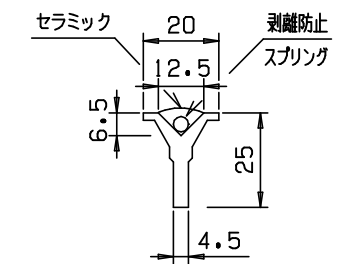
補助部材Yバー部詳細
