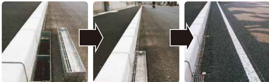
施工状況写真 (広島県)
