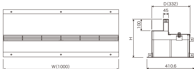
■サイドドレンゲッター 直用 (底板あり) 一体式
