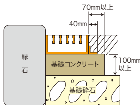
乗り入れ横断(新設)の場合
