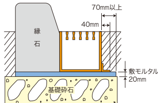
歩車道境界ブロック(新設)
