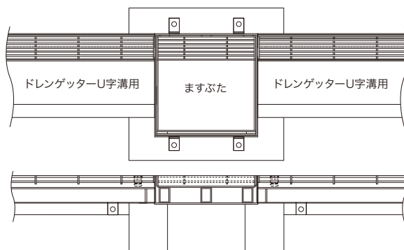
U字溝ドレンゲッターとますぶたの配置図
