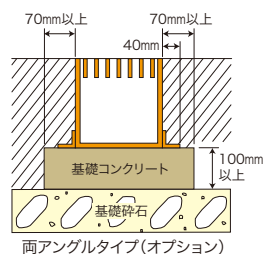
乗り入れ横断(新設)の場合
