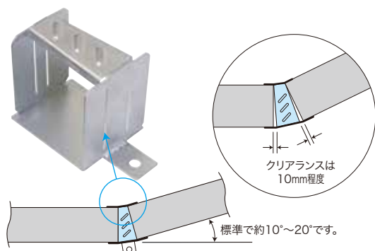
H-90用使用例
