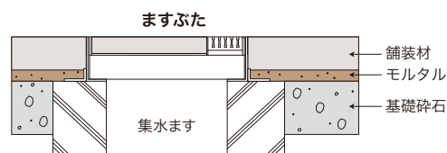
ステンレスドレン+化粧蓋 (愛知県)
