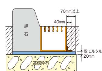
歩車道境界ブロック(新設)
