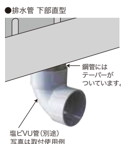
●排水管 下部直型
