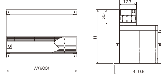
■サイドドレンゲッター専用 泥溜マス
