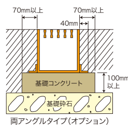
乗り入れ横断(新設)の場合
