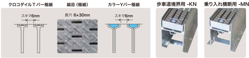
TADJF-3TT-10W20H-MN 可変用 H-200用 スキマ6 (山口県)
