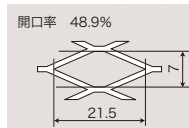
エキスパンド開口部（XS-33）
