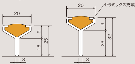
Yバーの寸法
