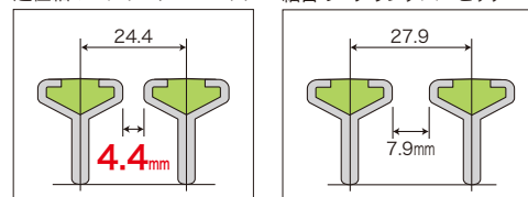
超極細のペアリングバーピッチ 細目のペアリングバーピッチ
