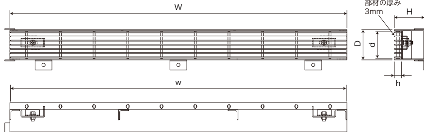
ステンレス製ドレン H-250特 スライドロック (愛知県)
