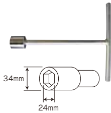
M16用ボックスレンチ 本体 普通目・細目固定用 価格(個)3,800円
