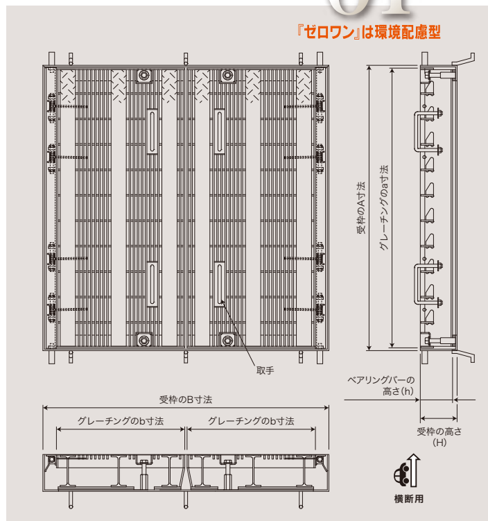
IBグレーチングボルト固定タイプ
