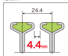
超極細のベアリングバーピッチ
