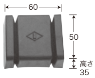
CAP-L 価格(個)550円 (普通目 H50~100用)
