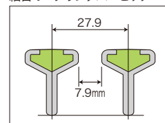
細目のベアリングバーピッチ
