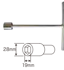
M12用ボックスレンチ 本体 普通目固定用(H25) 価格(個)2,700円
