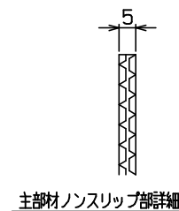
主部材ノンスリップ部詳細
