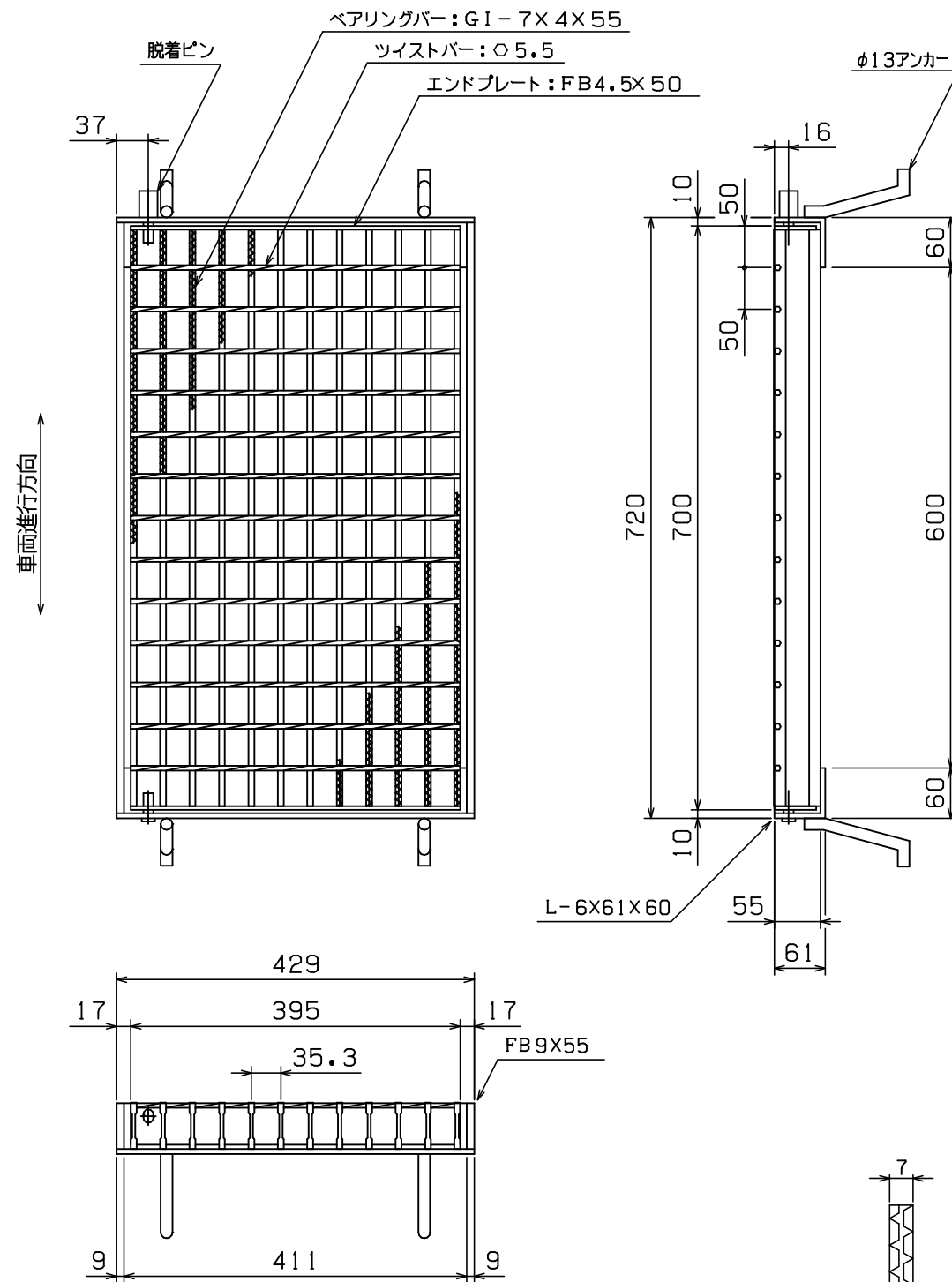
主部材ノンスリップ部詳細
