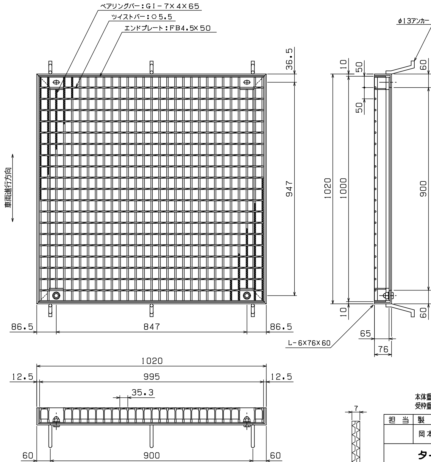
主部材ノンスリップ部詳細
